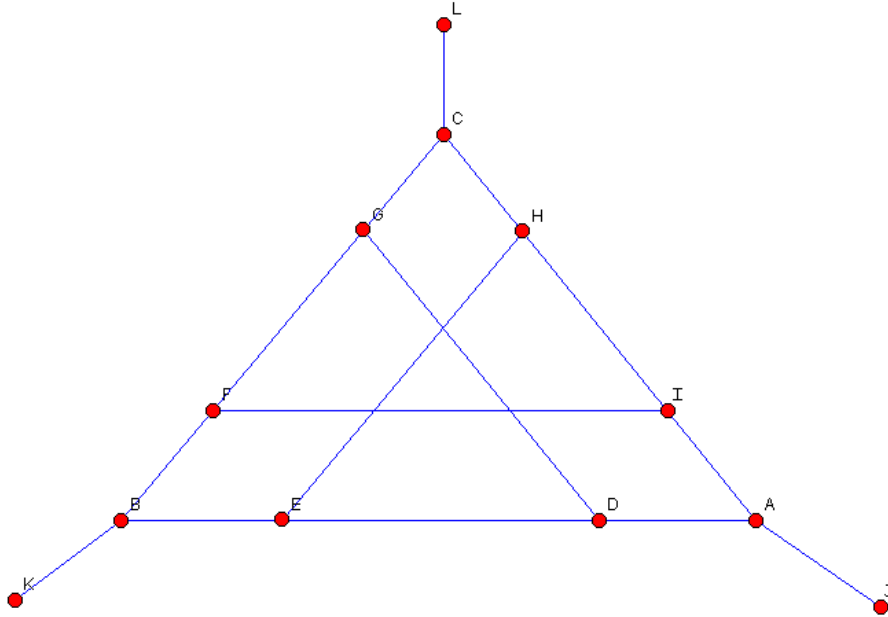
Figura 2: Menor grafo conhecido cuja interseção de todos os caminhos mais longos é vazia
