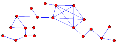
Grafo de blocos
