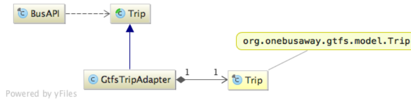
Figura 8: Uso do padrão adapter . As funcionalidades da classe org.onebusaway.gtfs.model.Trip podem ser aproveitadas devido à existência do adapter .
