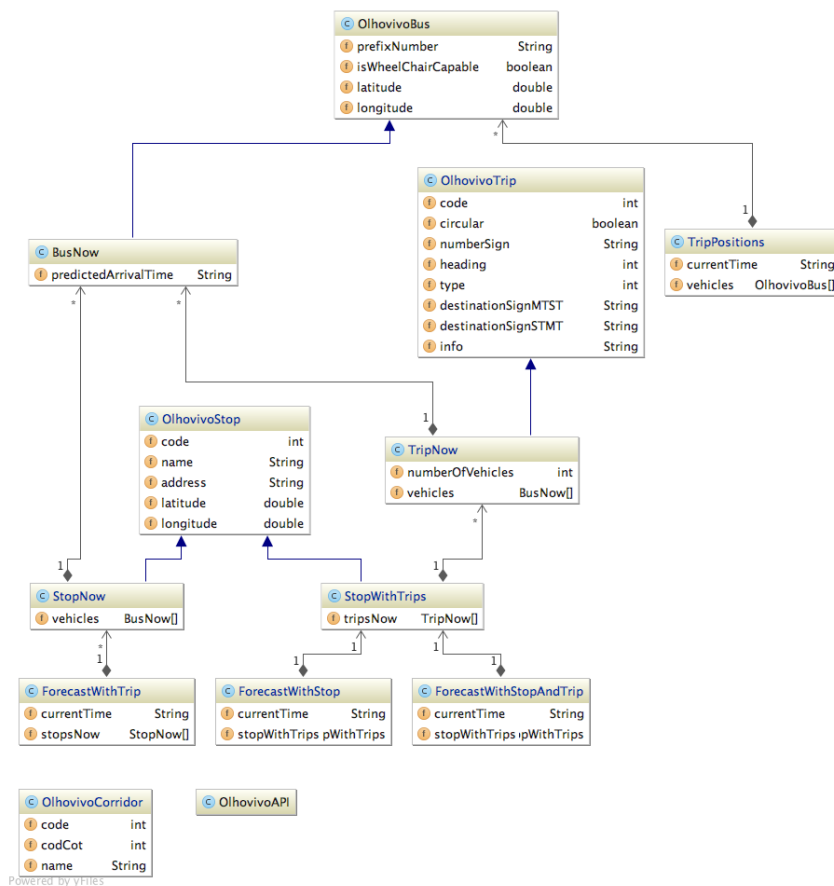
Figura 18: Pacote olhovoapi. Mostrando apenas os atributos das classes. Classes criadas apenas para poder usa a biblioteca Jackson para lidar com as respostas JSON.
